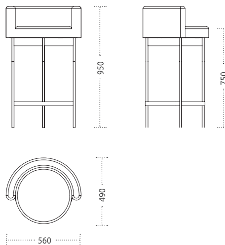
Sgabello alto High stool
